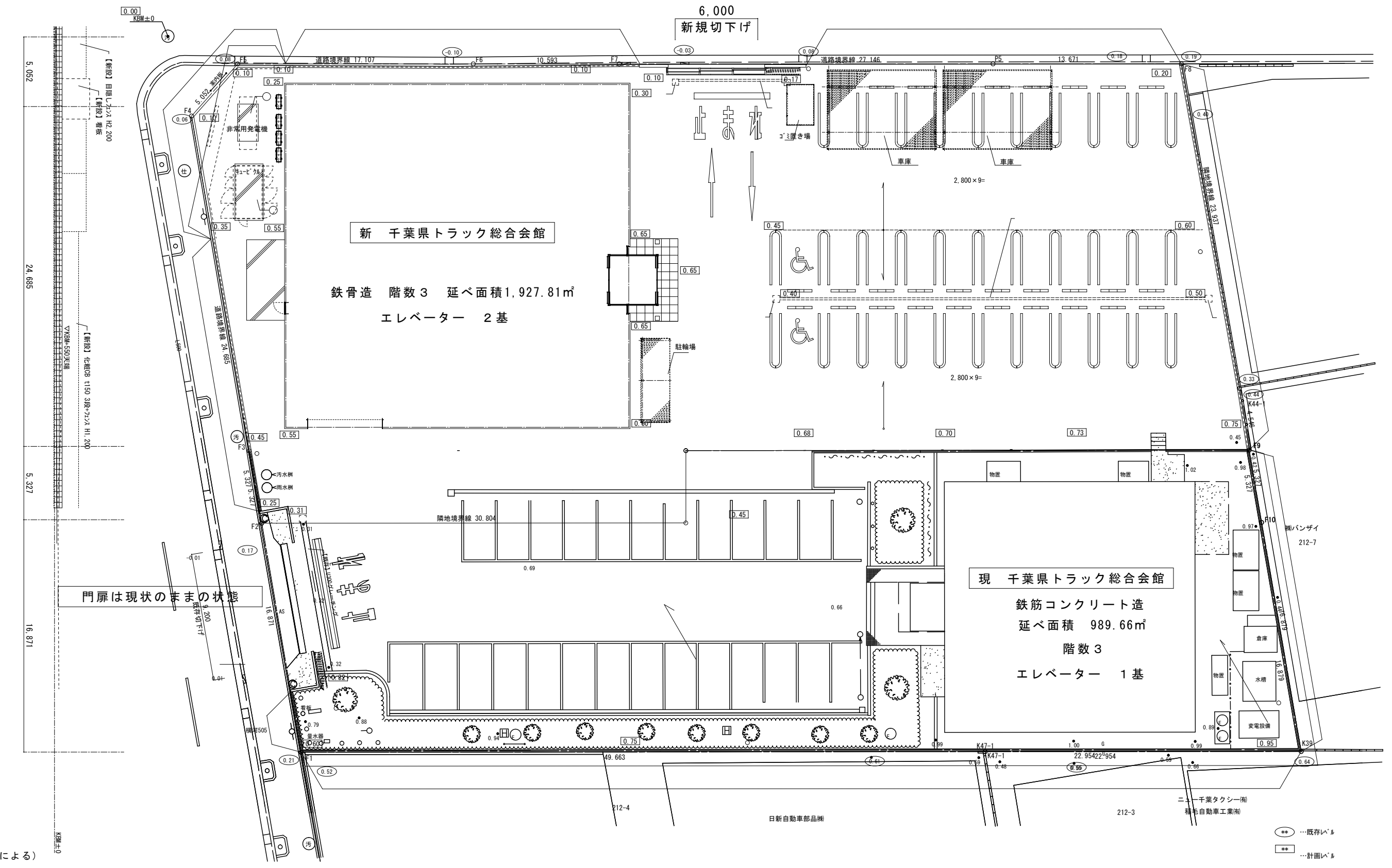
新千葉県トラック総合会館の事務所引越等業務実施時の配置図
